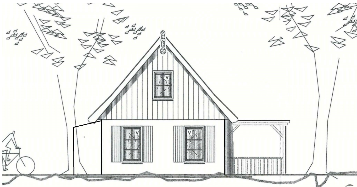
Voorgevel
